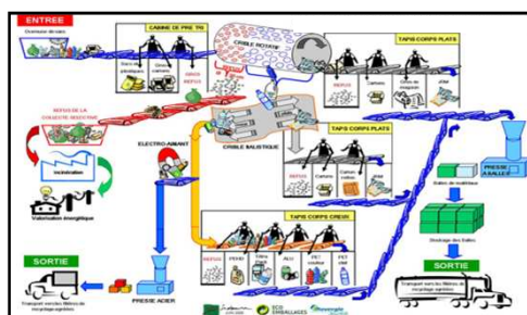
SCHEMA DE PRINCIPE DE LA CHAINE DE TRI
